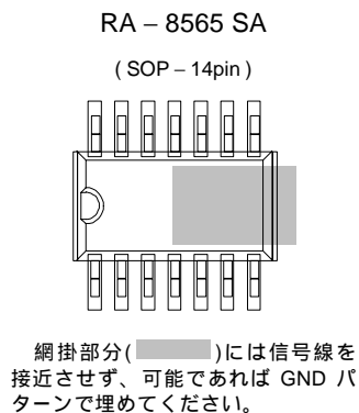
図 1 : GND パターン例
