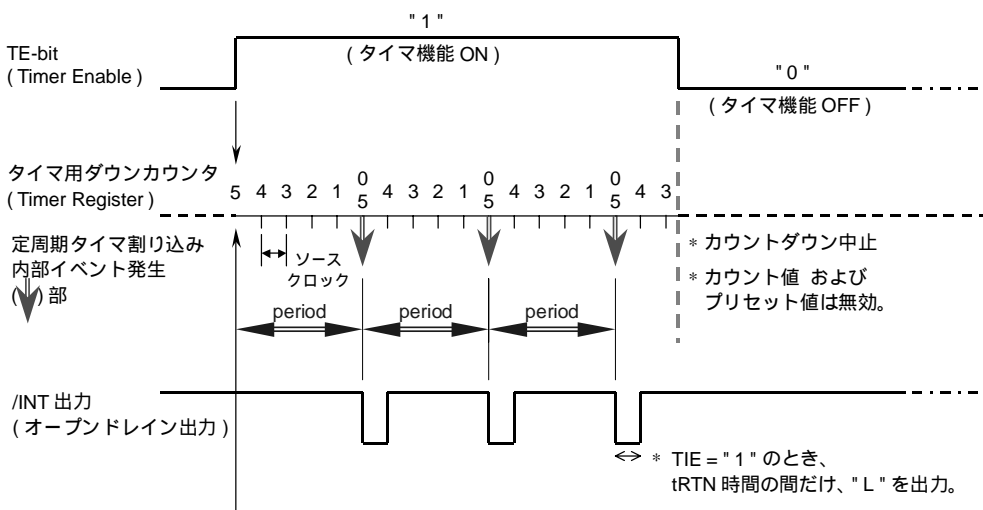
[繰り返し割り込みモード時 且つ プリセット値 5 (05h)] とした場合の動作例
