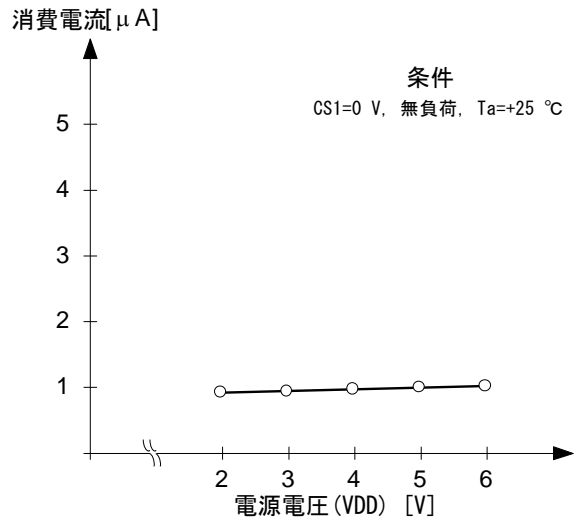
(3) 消費電流電圧特性例
