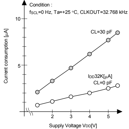
(3-2) 非アクセス時 消費電流 (ii) CLKOUT=32.768 kHz 時
