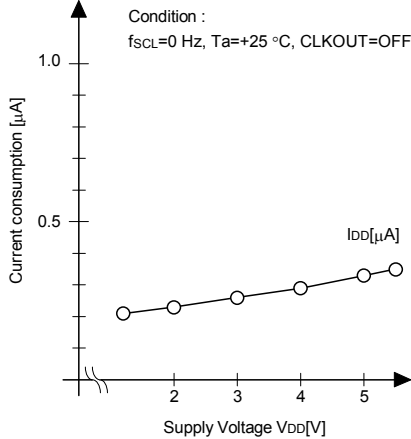
(3-1) 非アクセス時 消費電流 (i) CLKOUT=OFF 時
