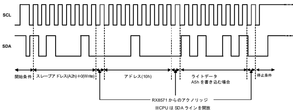
① アドレス指定の読みだし波形 アドレス 10h に A5h を書き込む場合
