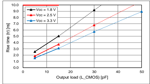
20 % - 80 %V CC , T use = +25 °C, Output load Char.
