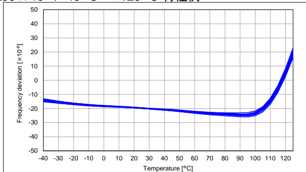
\pm 50 \times 10^{-6} / -40 \text{ }^\circ\text{C} \sim +125 \text{ }^\circ\text{C} 特性例
