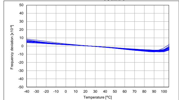
\pm 20 \times 10^{-6} / -40 \text{ }^\circ\text{C} \sim +105 \text{ }^\circ\text{C} 特性例
