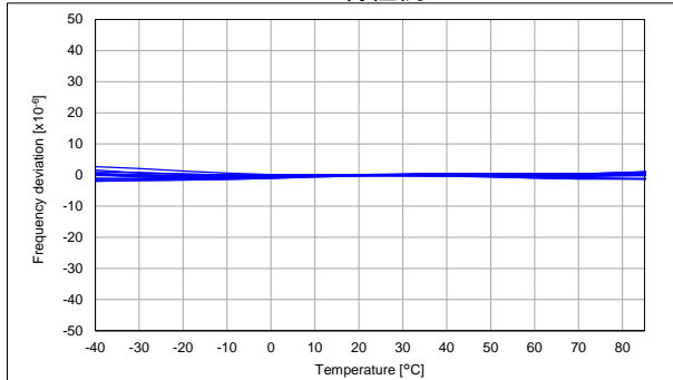
\pm 15 \times 10^{-6} / -40 \text{ }^\circ\text{C} \sim +85 \text{ }^\circ\text{C} 特性例
