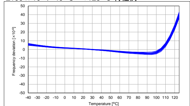
\pm 100 \times 10^{-6} / -40 \text{ }^\circ\text{C} \sim +125 \text{ }^\circ\text{C} 特性例
