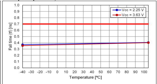
Output option:B, Fall Time
