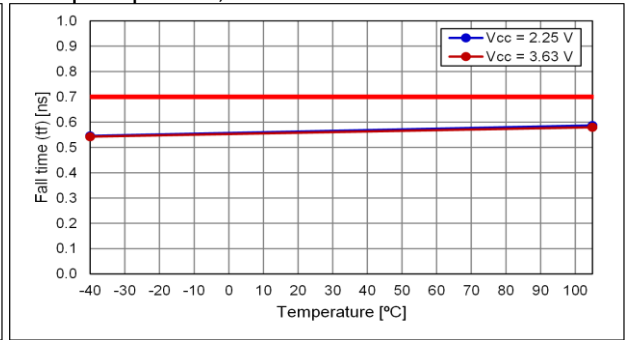
Output option:A, Fall Time
