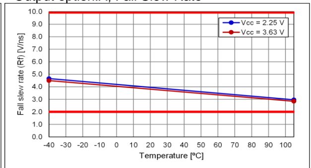
Output option:A, Fall Slew Rate
