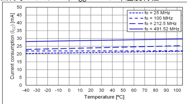
出力オプション:A, V_{CC} = 2.25 V, 温度特性
