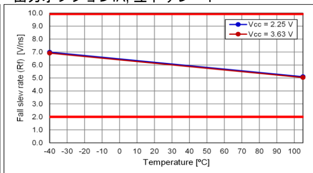
出力オプション:A, 立下りレート
