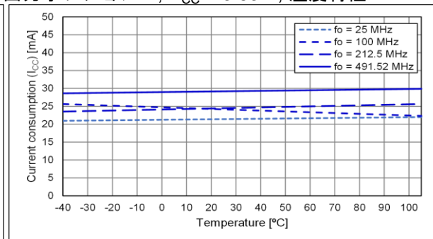
出力オプション:A, V_{CC} = 3.63 V, 温度特性
