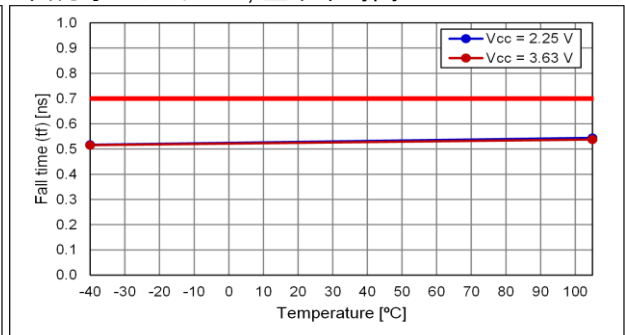
出力オプション:B, 立下り時間
