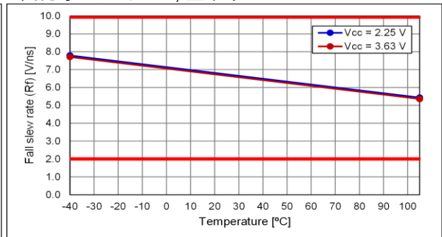
出力オプション:B, 立下りレート
