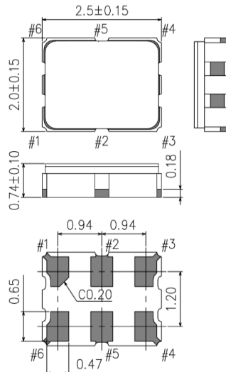
SG2520HHN
