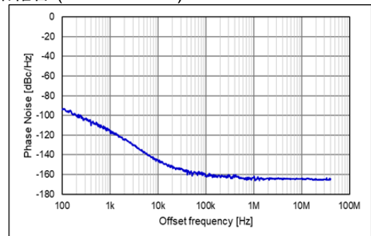
位相ジッタ (12 kHz ~ 20 MHz): 60 fs Typ.
