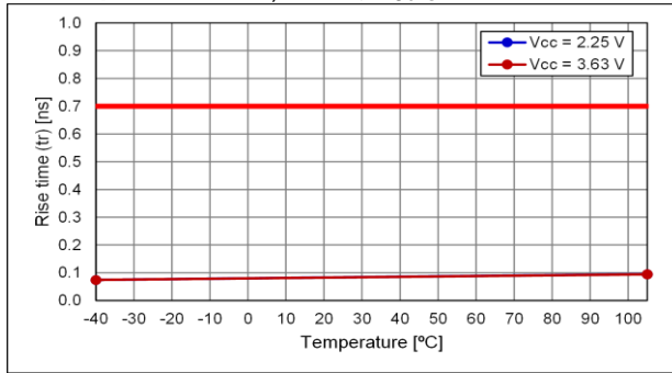
出力オプション:A, 立上り時間
