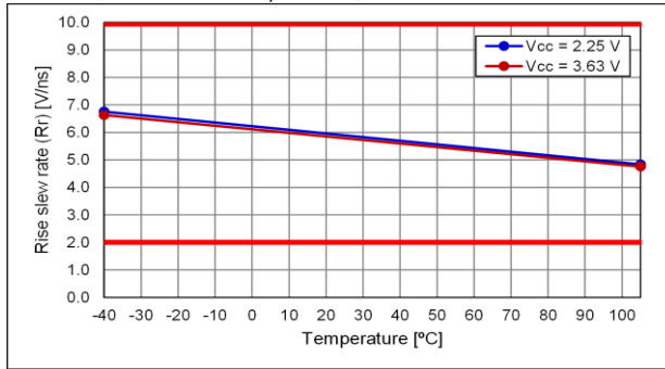
出力オプション:A, 立上りレート
