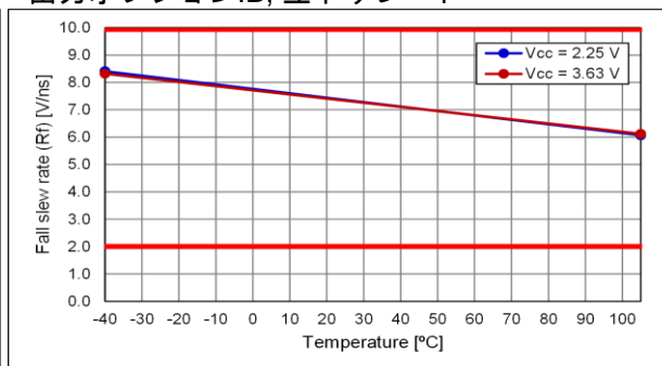
出力オプション:B, 立下りレート
