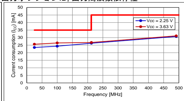
出力オプション:B, 出力周波数依存性
