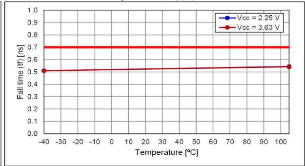
出力オプション:A, 立下り時間
