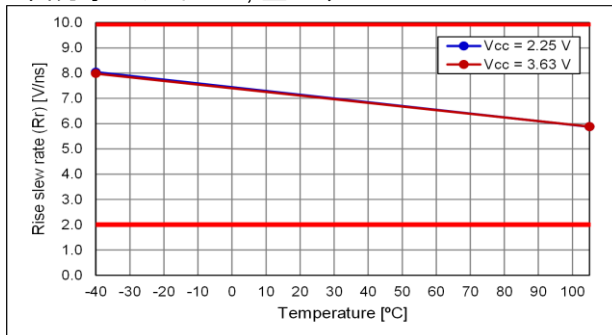
出力オプション:B, 立上りレート
