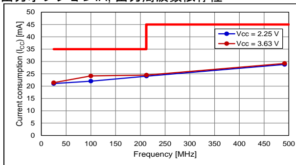
出力オプション:A, 出力周波数依存性
