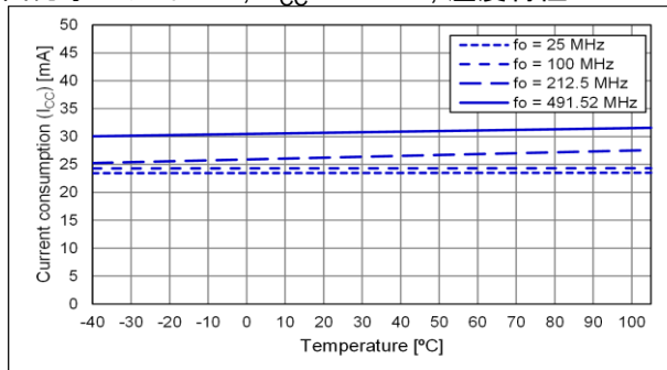
出力オプション:B, V_{CC} = 2.25 V, 温度特性
