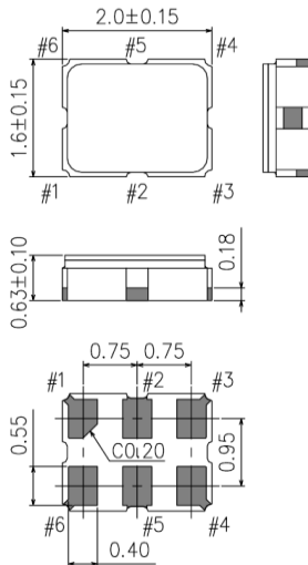
SG2016HHN
