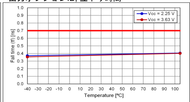
出力オプション:B, 立下り時間
