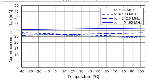
出力オプション:B, V_{CC} = 3.63 V, 温度特性
