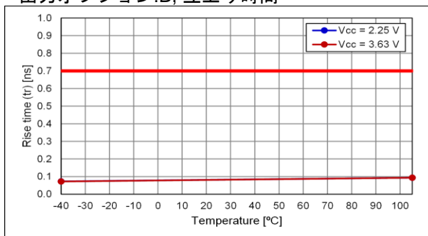
出力オプション:B, 立上り時間
