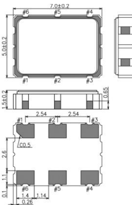
SG7050VEN
