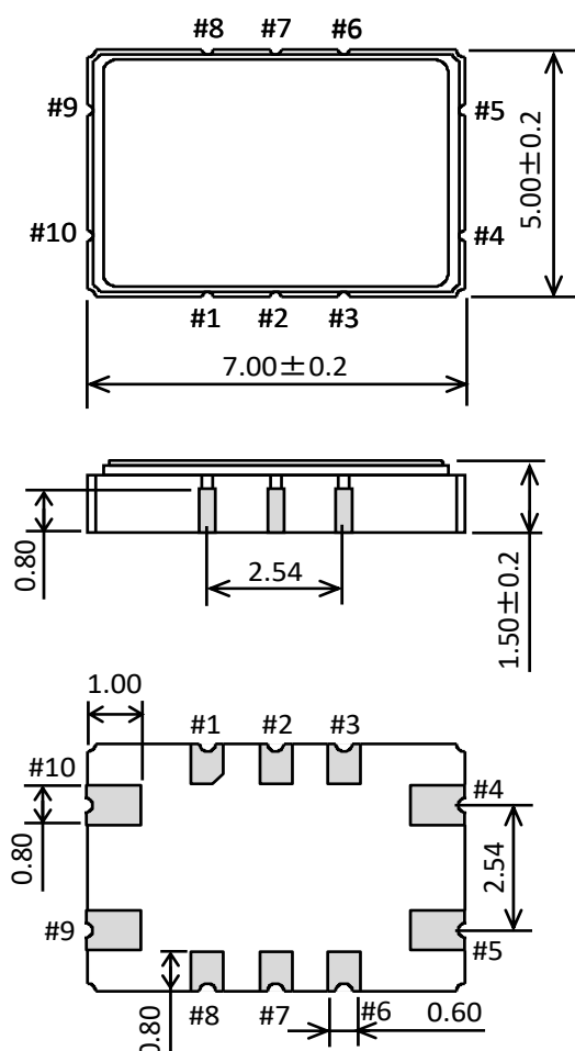
[ 8 ] 外形寸法図 単位: mm
