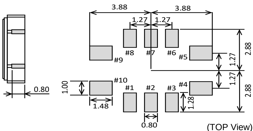
[ 9 ] フットプリント(推奨) 単位: mm
