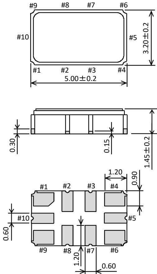
[ 8 ] 外形寸法図 単位: mm
