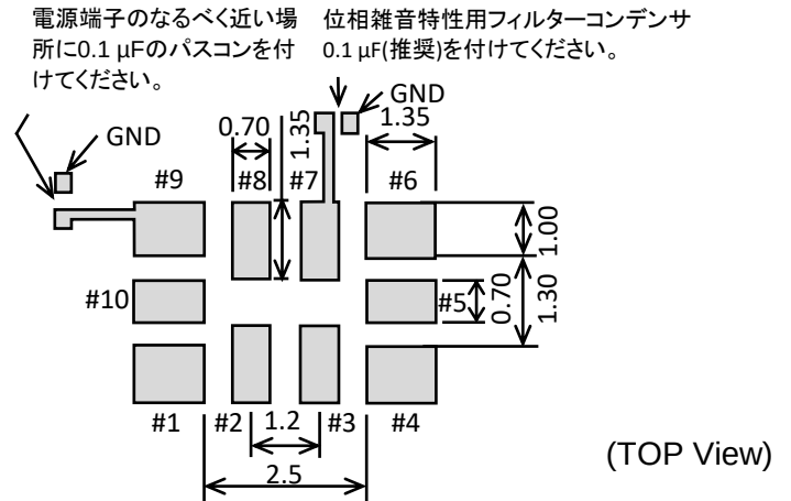
端子説明
