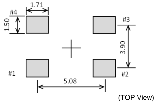
[ 9 ] フットプリント(推奨) 単位: mm
