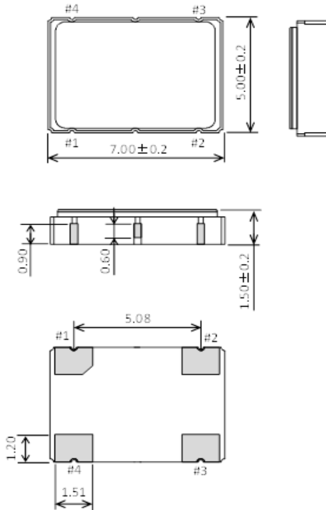
[ 8 ] 外形寸法図 単位: mm
