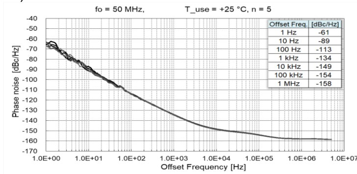
12) fo = 50 MHz
