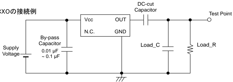
(2)VC-TCXOの接続例
