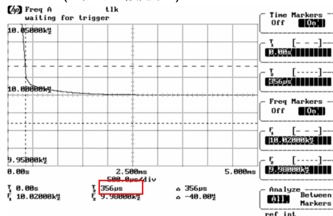
20MHz (フィルター設定なし)
