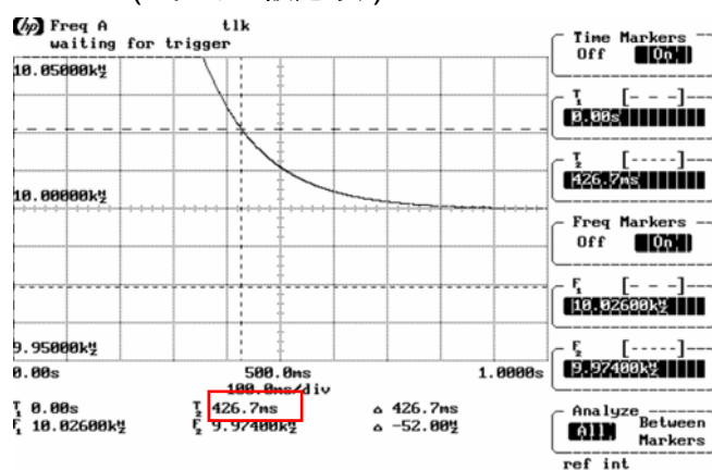
26MHz (フィルター設定あり)
