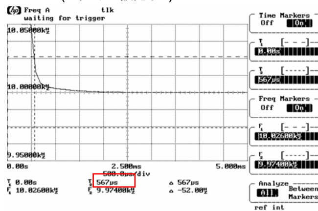
26MHz (フィルター設定なし)
