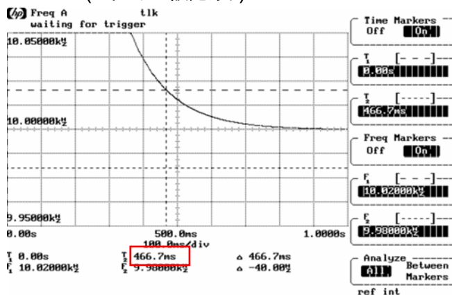
20MHz (フィルター設定あり)
