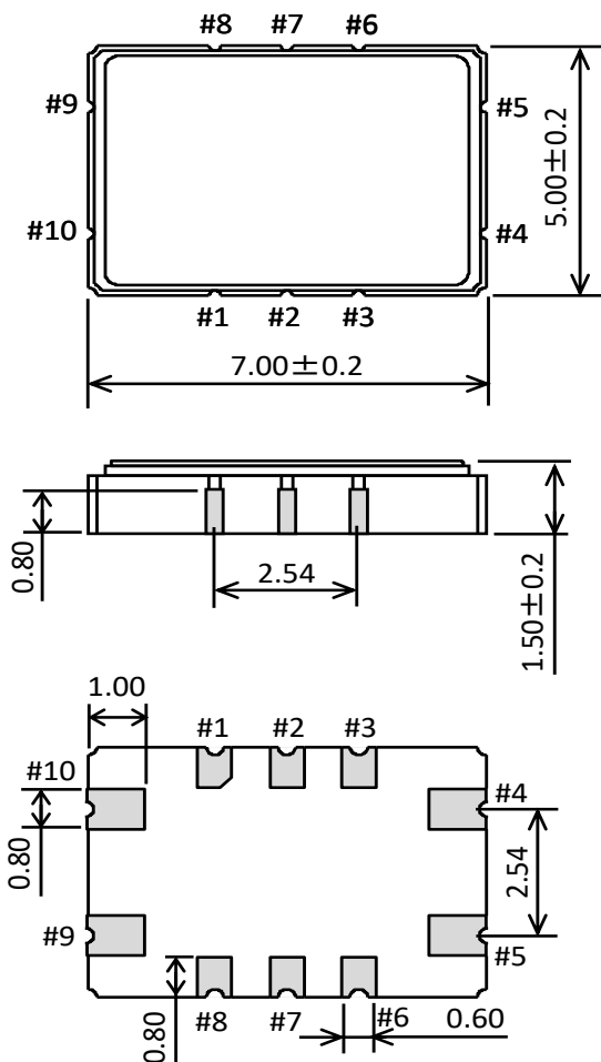
[ 8 ] 外形寸法図 単位: mm
