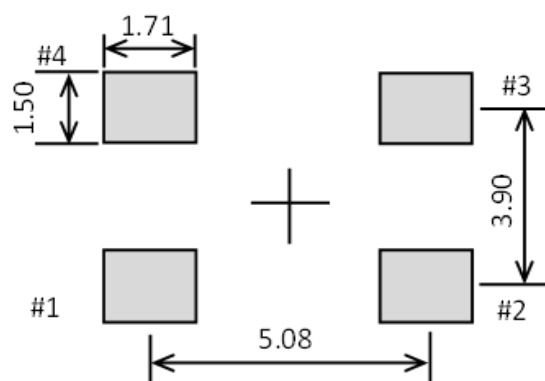
[ 9 ] フットプリント(推奨) 単位: mm
