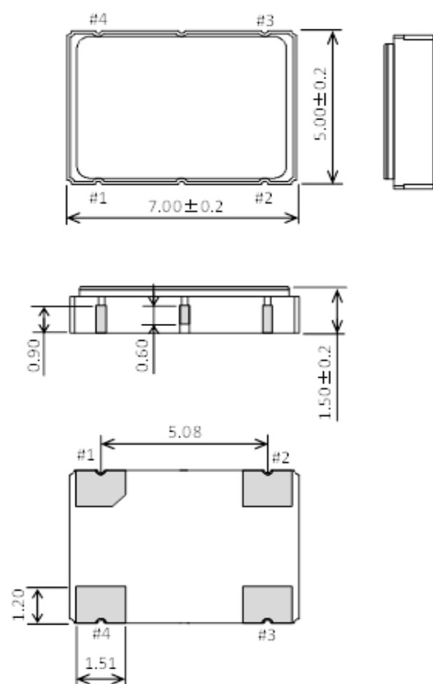
[ 8 ] 外形寸法図 単位: mm
