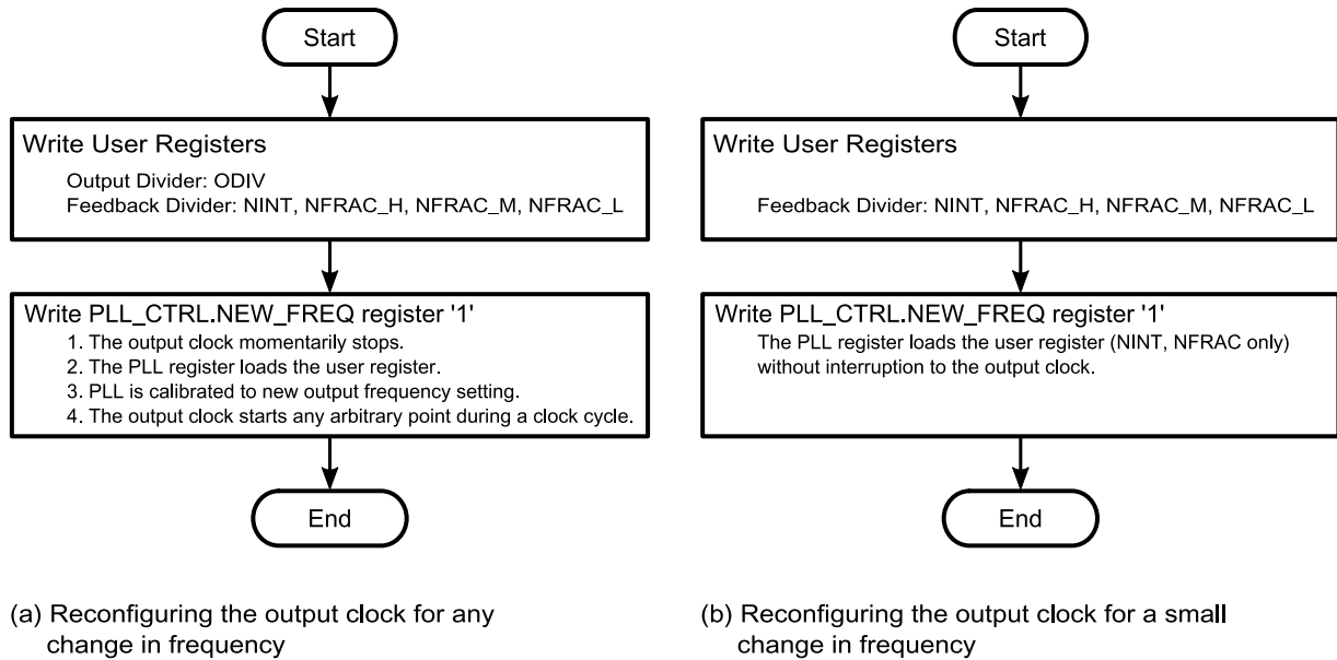
図 6.1 周波数の設定手順
