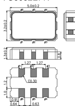
VG5032EFN
