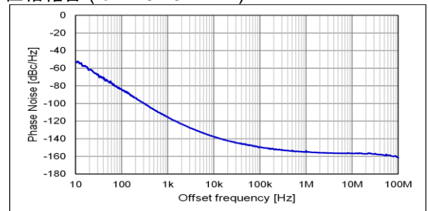
位相雑音 (fo = 491.52 MHz)
