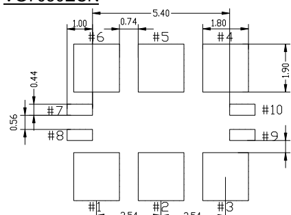
VG7050ECN
