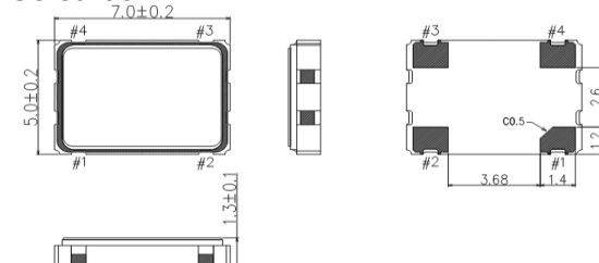
SG-8018CA
