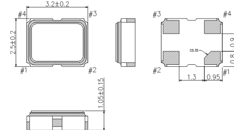
SG-8018CA
